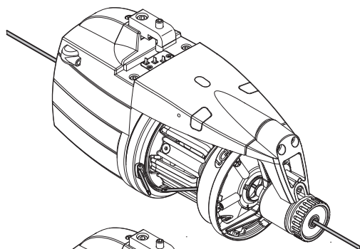
INFILAGGIO PARZIALE
