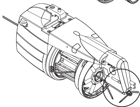
INFILAGGIO COMPLETO VERSIONE ATTIVO
